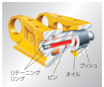
▲ピンのリンク抜けを防ぐリテーニングリングをピン部に装着。
