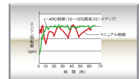
ARC制御とマニュアル制御とのエンジン回転数の変動比較
