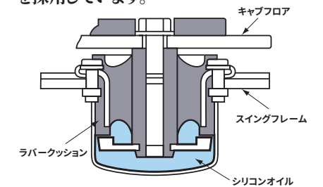
キャブマウントに採用の新型ビスカスマウント
