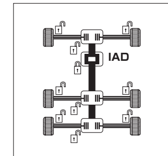
インターアックスルデフ (IAD) のみロック
