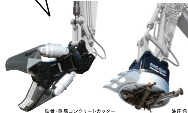
鉄骨・鉄筋コンクリートカッター ガジラDSカッター [タグチ工業]
